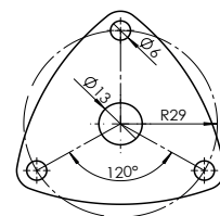
Flansch mit Dichtung 20.045
