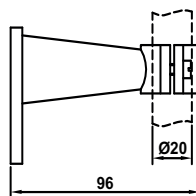
Wandkonsole 20.009
