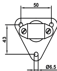
Wandkonsole 20.009
