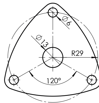
Bohrbild Befestigungsflansch
